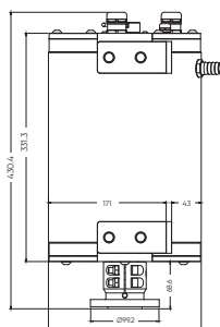
zijaaanzicht
