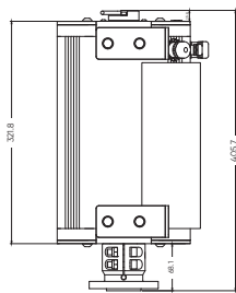
zijaaanzicht
