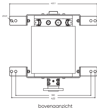
bovenaanzicht
