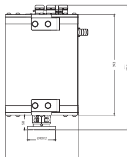
zijaaanzicht
