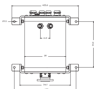
bovenaanzicht
