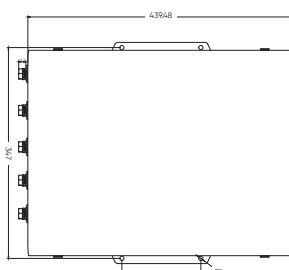
bovenaanzicht
