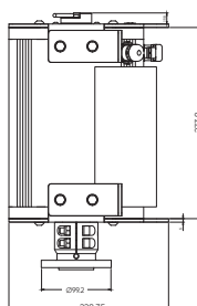
zijaaanzicht
