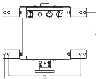
bovenaanzicht
