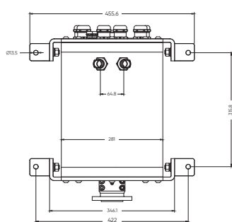
bovenaanzicht
