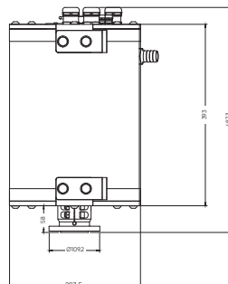
zijaanzicht
